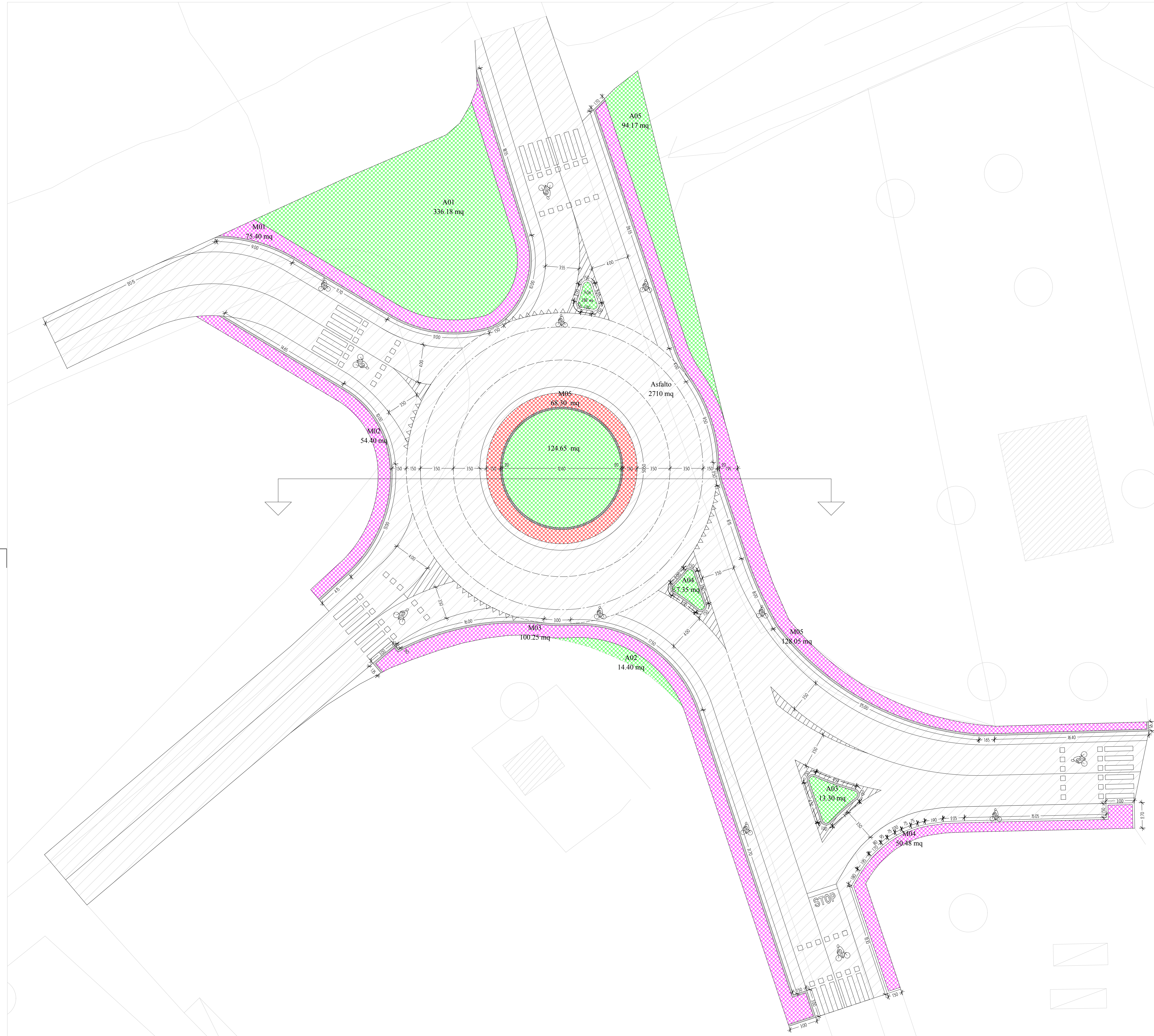
PLANIMETRIA QUOTATA SCALA 1:200
